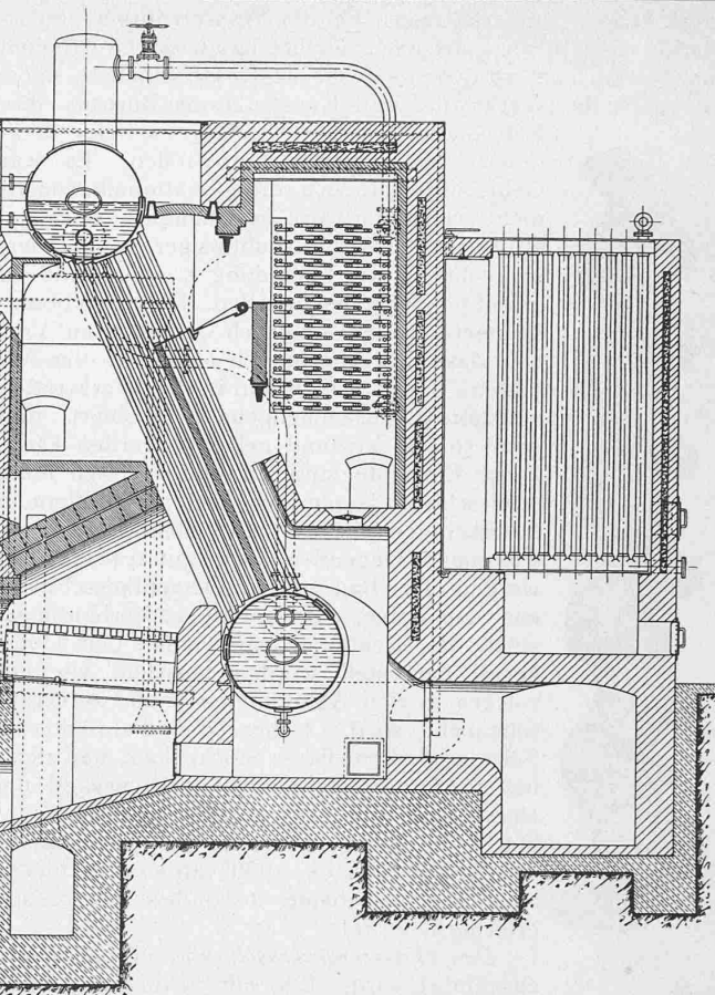
Abb. 12. Einbündel-Garbe-Kessel, bis 200 m 2 Heizfläche. — Masstab 1:100.
