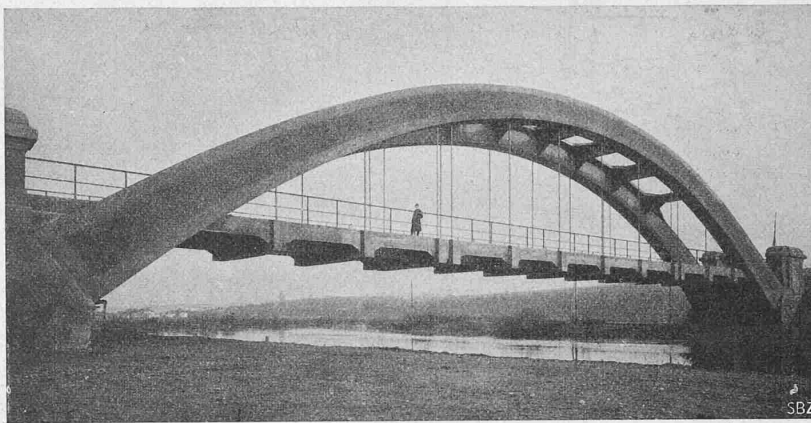
Abb. 1. Eisenbahnbrücke bei Heringen, erbaut 1910 durch Christiani & Nielsen.
