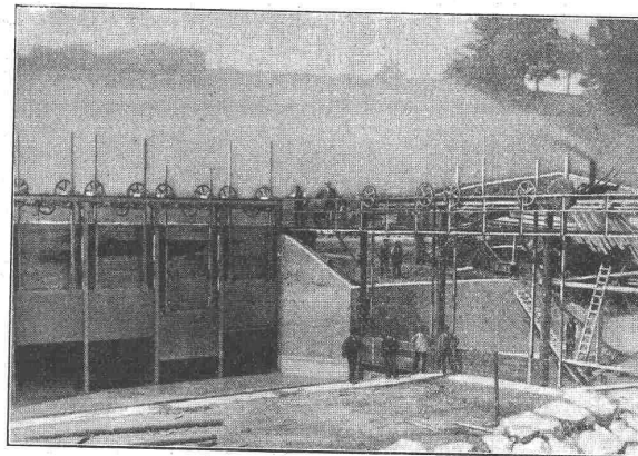
Komplette Fallenzüge für Rheinkorrektion Rorschach. Eisengewicht 52,3 Tonnen.
