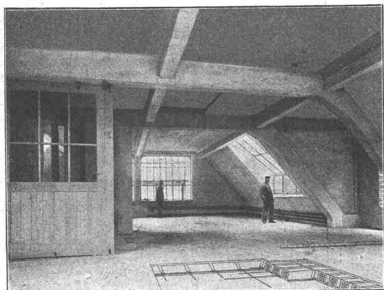
Industriebau in Steineisenbetonkonstruktion, ausgeführt 1909/10, zur Zeit im Bau.
