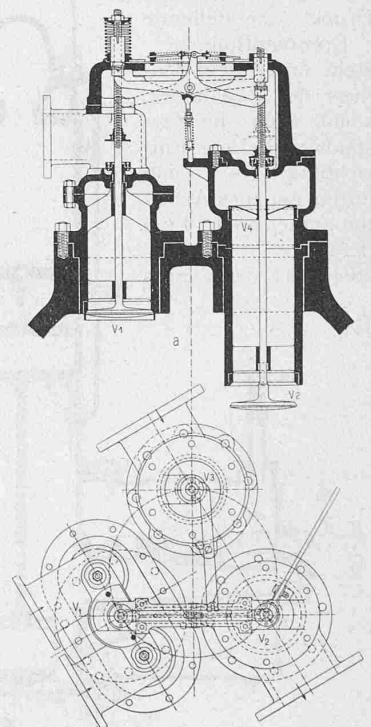
Abb. 57. Ventilkopf. — Etwa 1:20.
