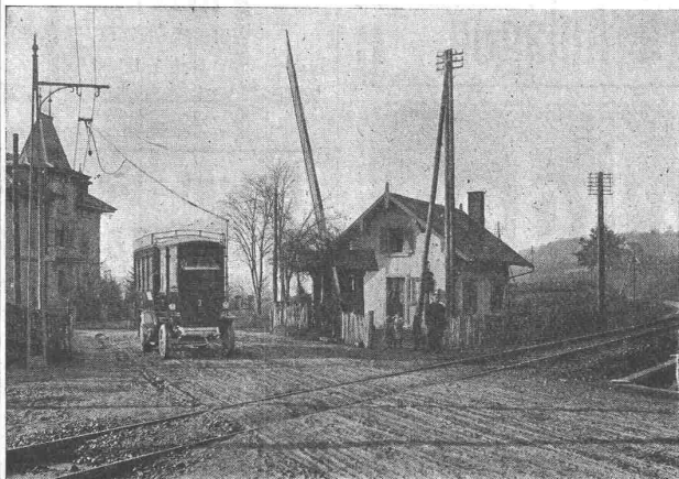
Linie Fribourg-Posieux, Niveau-Uebergang in La Glâne.
