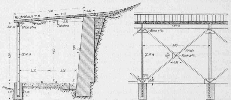
Abb. 56. Schneeschutzgalerie mit Bohlenabdeckung. — 1 : 150.
