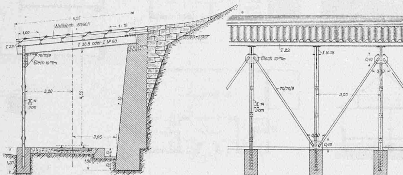
Abb. 55. Schneeschutzwand mit Wellblechabdeckung. — Masstab 1:150.
