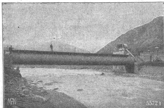
Walzenwehr in der Trisanna bei Landeck in Tirol. 1,10 m Stauhöhe, 14,00 m Länge.
