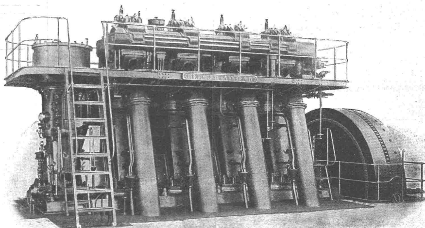
1500 PS Sulzer Diesel-Zweitaktmotor
