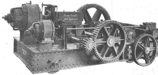
Elektrische Kranwinde von 120 Tonnen Tragkraft.
