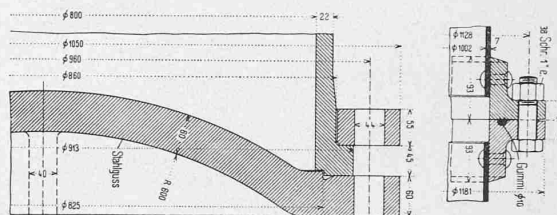
Abb. 17. Abschlussdeckel.
