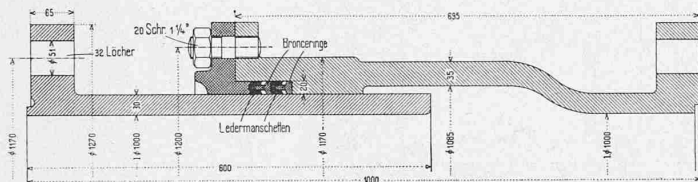
Abb. 16. Längsschnitt der Expansion — Masstab der Details 1 : 10.
