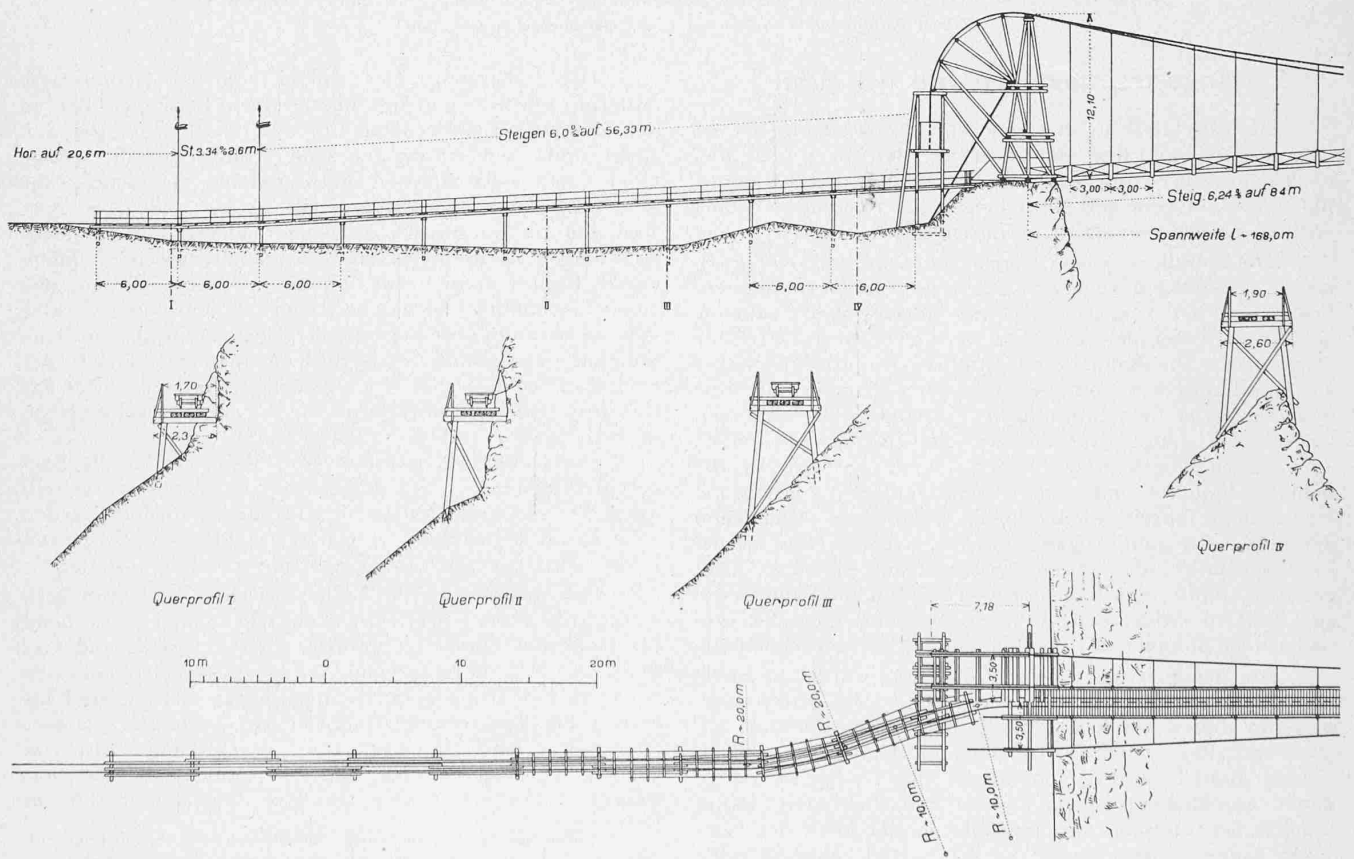
Abb. 4. Rechtsufriges Brückenende mit Spannungsgewichten und Zufahrts-Lehnenviadukt 1 : 500, Querprofile 1 : 250.
