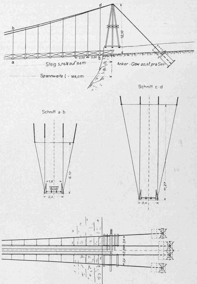
Abb. 5. Linksufriges Brückenende 1 : 500, Schnitte 1 : 250.
