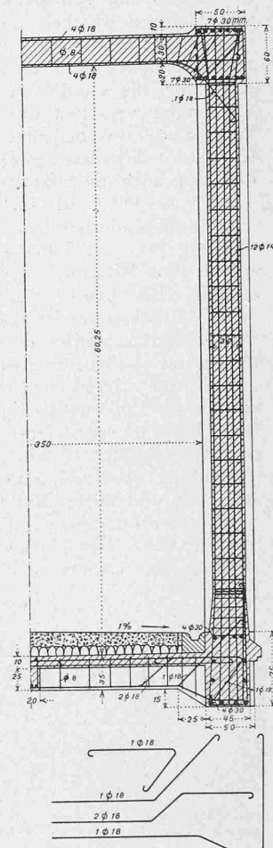
Abb. 4. Querschnitt 1 : 60.
