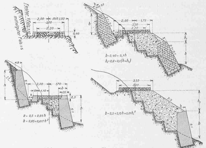
Abb. 12. Normalprofile. — 1 : 200.
