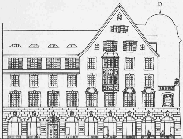
Abb. 2. Wettbewerbs-Entwurf. — Fassade an der Poststrasse, Masstab 1:400. — Abb. 3. Ausgeführte Fassade.
