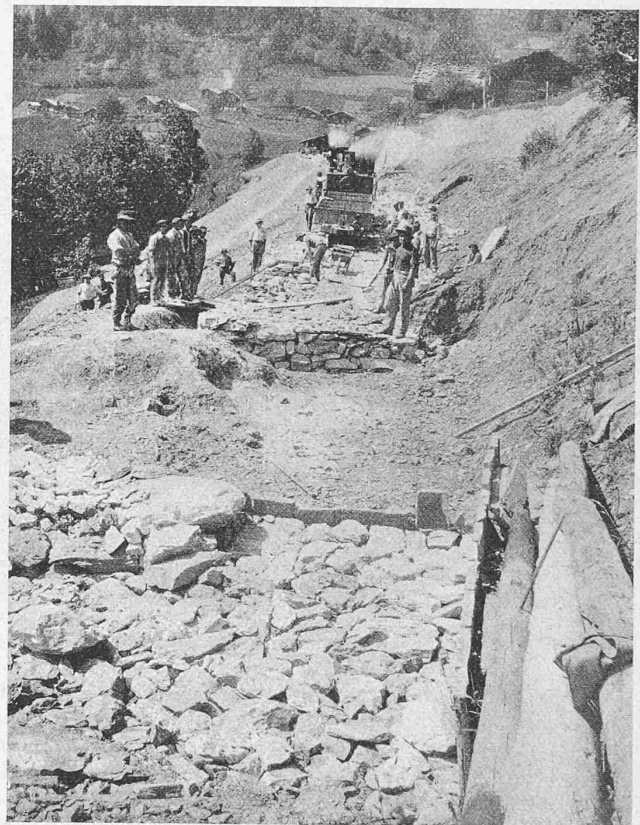
Abb. 33. Bahnkörper mit Sickerschächten bei Km. 3,0.
