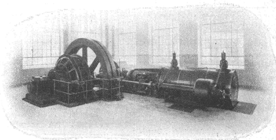
700 PS-Gleichstrom-Dampfmaschine im Guss- und Armaturwerk Kaiserslautern.
