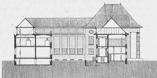
Längsschnitt Nord-Süd durch den Hof. — 1:800.
