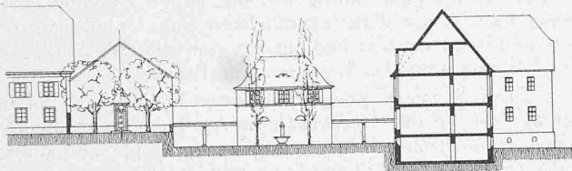
I. Preis. Entwurf Nr. 29 „Präludium“. — Querschnitt parallel zur Domstrasse (1:800) und Ansicht des Schulhauses vom Domplatz aus.
