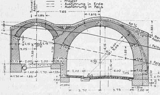
Abb. 10. Profiltypen der Bodensee-Toggenburgbahn. — Masstab 1 : 250.
