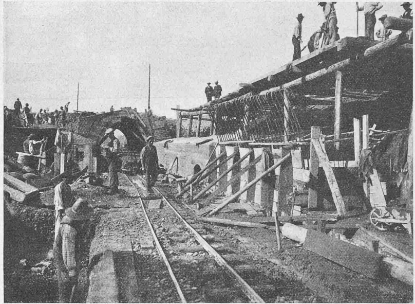
Abb. 14. Verlängerung des Taltunnels bei Herisau.
