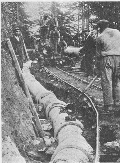
Abb. 12. Vergiessen der Siegwart-Röhren an der Intschi-Leitung.
