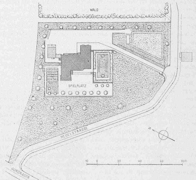
Abb. 1. Lageplan. — Masstab 1 : 2000.
