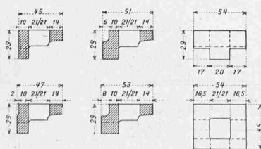
Abb. 5 Zahnstange; Abb. 6 Schienenprofil; Abb. 9 Klemmplättchen.
