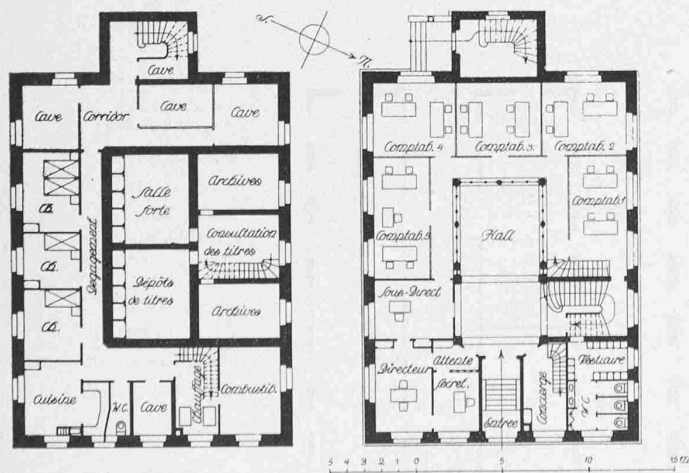
II. Preis ex æquo. Nr. 19. — Architecte Daniel Isoz, Lausanne. — Grundrisse und Schnitt 1 : 400.
