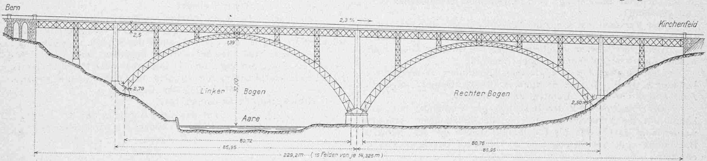
Abb. 1. Ansicht der Kirchenfeldbrücke in Bern, flussabwärts gesehen. — Masstab 1:1250.
