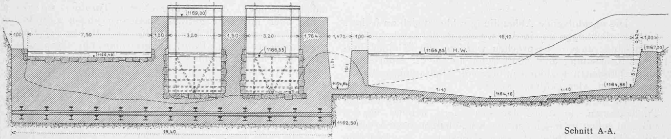
Schnitt A-A.
