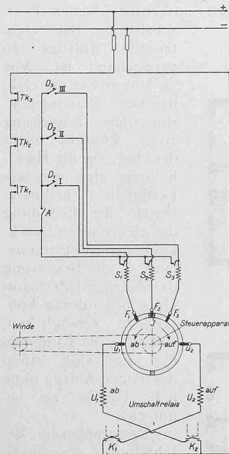
Abb. 1. Allgemeines Schaltungs-Schema einer Druckknopfsteuerung.
