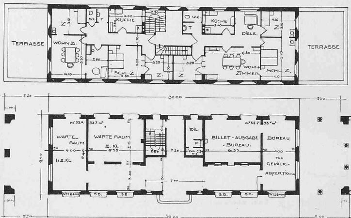
Entwurf für den Bahnhof Arosa. — II. Preis ex aequo. Motto „Schanfigg“. — Verfasser: Meier & Arter , Architekten in Zürich.
