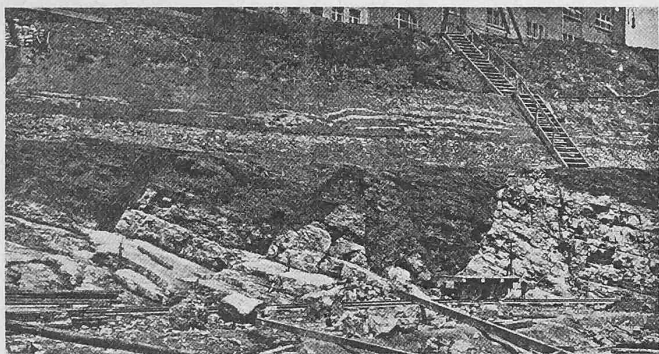
Abb. 6. Verwerfungen im rechtsufrigen Ablaufkanal.
