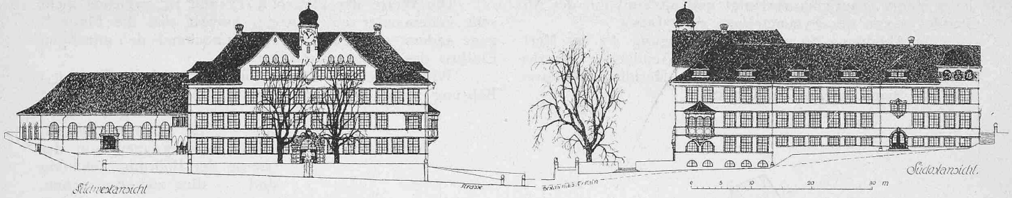
I. Preis. Entwurf Nr. 62. — Südwest- und Südostfassaden. — Masstab 1:800.
