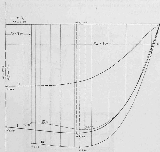
Abb. 36. Durchbiegung \Delta y in Funktion des Abstandes x von der Symmetrieaxe, für die Beispiele I, II, IX und IX v .
