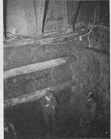
Abb. 20. Fundamentaushub unter der Schneide im Schwellen-Caisson 5a; Blick gegen den Pfeiler-Caisson IV. (Mai 1911) (Die Aufnahmen zu Abb. 17 und 20 stammen von Herrn Ing. Hermann Gamper, Bauführer der Unternehmung Cd. Zschokke.)
