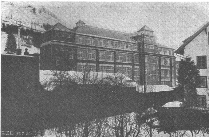
Mechanische Weberei Zell A.-G. in Zell Hochbau und Shedbau in Eisenbeton. Ausgeführt 1907. Aussenansicht des Hochbaues.
