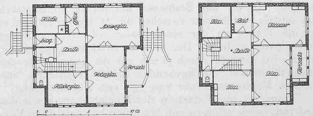
Abb. 8 und 9. Grundrisse. — 1:400.
