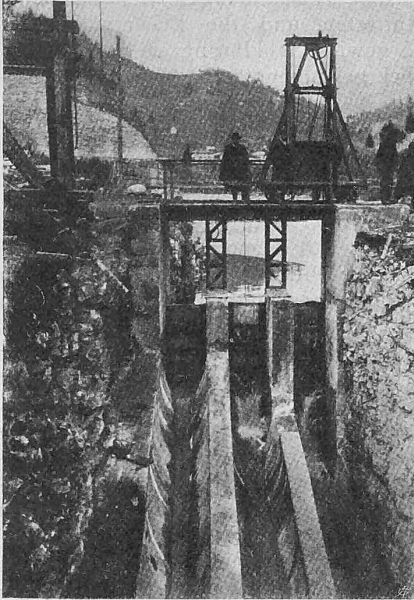
Abb. 6. Flössrinnen-Einläufe.
