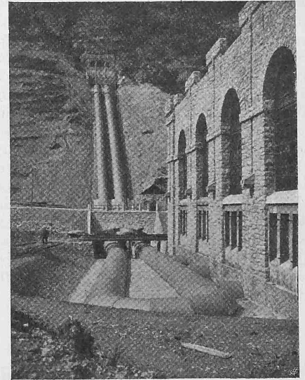
Abb. 17. Druckleitung 2 \times 1,9 m \phi .
