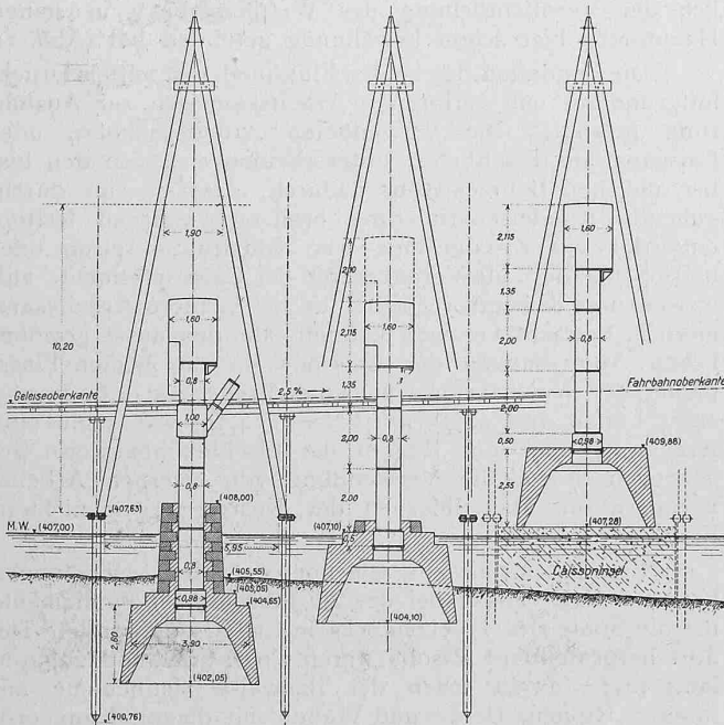
Abb. 2. Charakteristische Caissonlagen. — 1 : 250.
