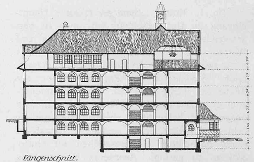
Langenschnitt.
