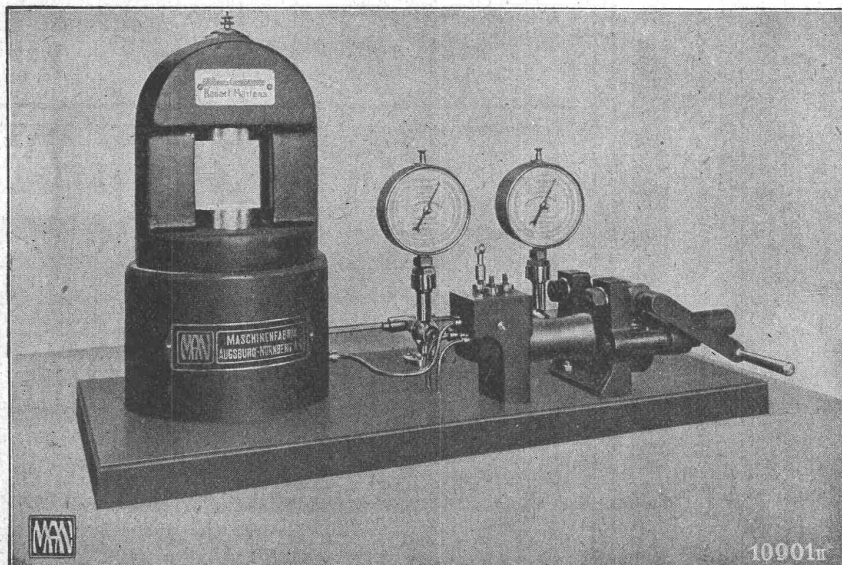
1 M. A. N.-Zementprüfer, System Martens, 50000 kg Tragkraft.
