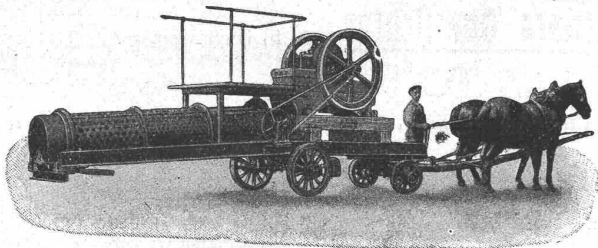
Ortsfeste und fahrbare Sandmählanlagen. Automobilsteinbrecher, Schotteranlagen auf Automobilen.
