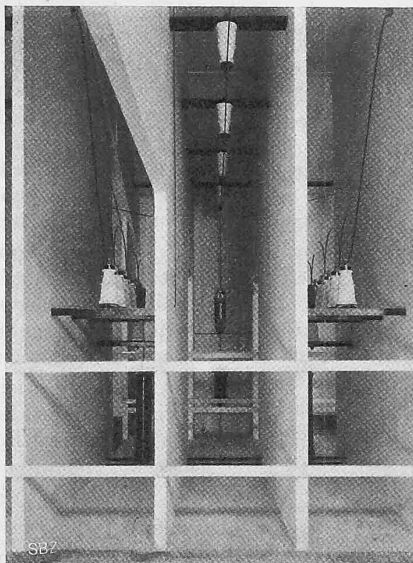
Abb. 55. Ueberspannungsschutz 44000 Volt.
