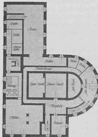
Grundrisse 1: 600. Lageplan 1: 1000.
