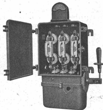
Schaltkasten mit III-poligem Oelschalter und Sicherungen
