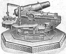
Modell einer Rohrücklauf-Haubtze. Gel. für die Kaiserl. chinesische Regierung.
