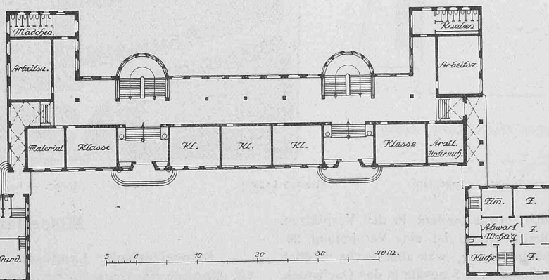
III. Preis. Motto „Bölle.“ Grundrisse vom Keller, Erdgeschoss und I. Stock. Masstab 1:800.
