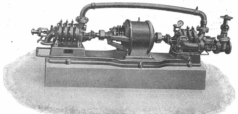
Zentrifugalpumpen
