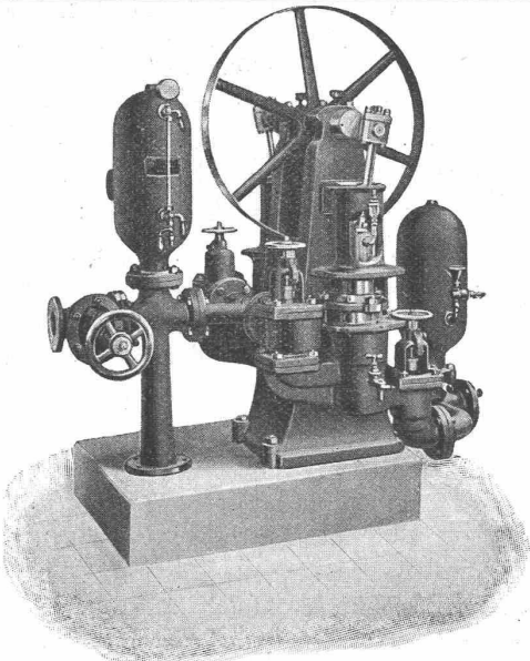
Kolbenpumpen
