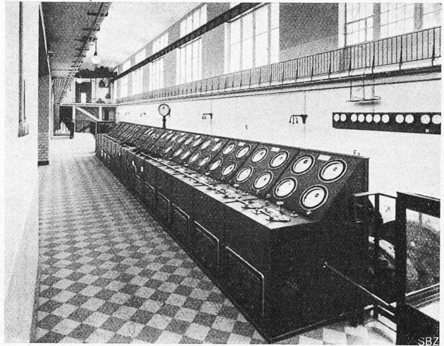
Abb. 57. Maschinen-Schaltpult.
