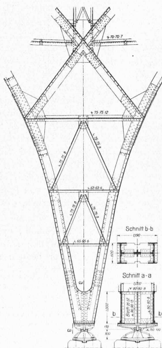
Abb. 41. Binderfuss. — 1:100.
