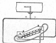
Druckmessermesser nach Krell mit Staurohr Dr. Brabbée.
