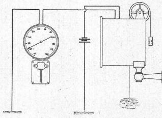
Wasserstandsmelder. Elektromagnetisches System.
