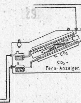
Mit ständiger Anzeige durch Flüssigkeitsfaden.
