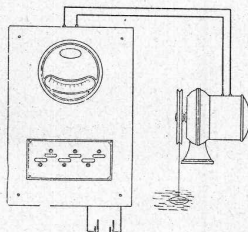
Wasserstandsmelder. Kontrollapparat.
