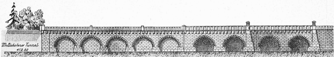
Abb. 9. Längsschnitt durch das Südende der Station Enge, Ansicht der Sihlbahn-Einmündung unter der verlegten Grütlistrasse (vergl. Abb. 8, S. 276). — 1:500.
