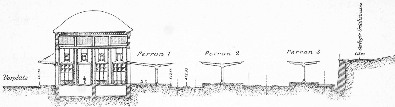
Abb. 6 (links nebenan S. 276) Querschnitt durch Nordende, Abb. 7 durch die Mitte der Station Enge. — Masstab 1:500.
