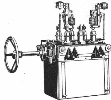
Automatiche Oelschalter
