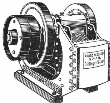
Backenbrecher
