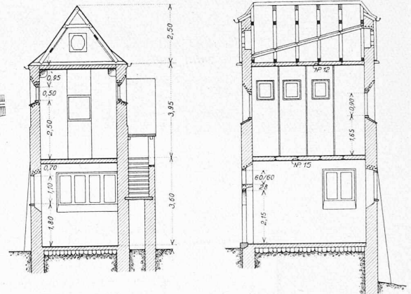
Abb. 2. Transformator-Häuschen Zuoz. — 1 : 200.
