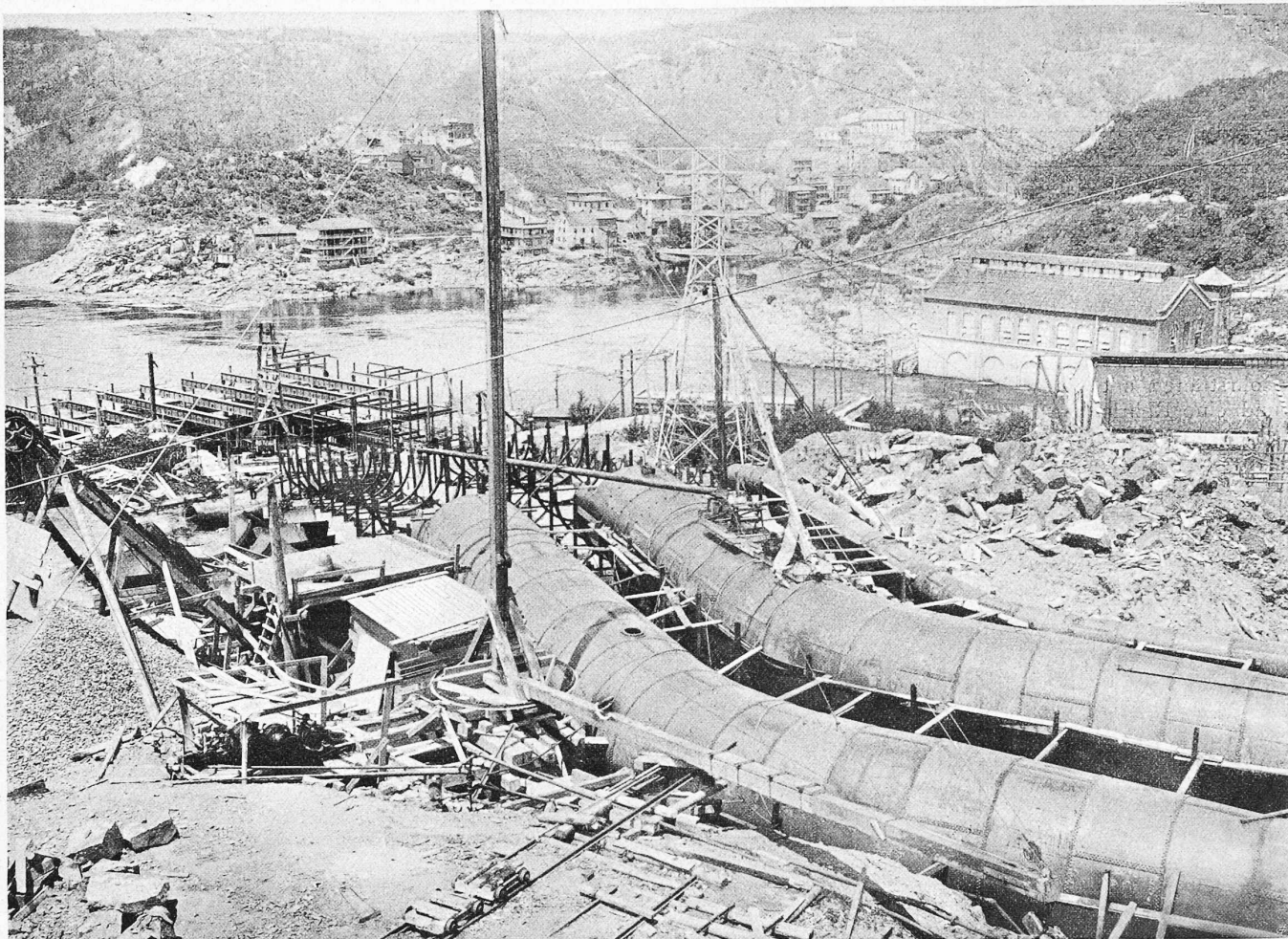
Abb. 13. Blick vom Wasserschloss nach N.-W., auf Rohrleitungen und Zentrale IV im Bau.
